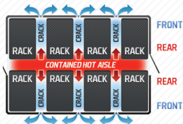
Модульная система охлаждения с изоляцией горячего коридора и рядным охлаждением
